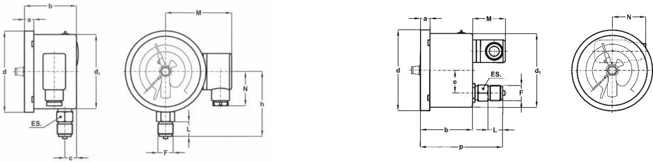
A - ПРИСОЕДИНЕНИЕ СНИЗУ
