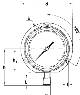
A - ПРИСОЕДИНЕНИЕ СНИЗУ
