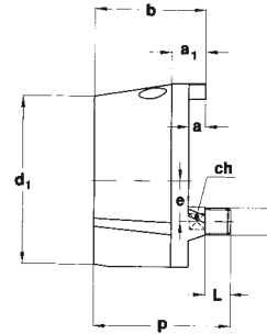
D - ПРИСОЕДИНЕНИЕ СЗАДИ, ТОЛЬКО ДЛЯ СТАНДАРТНОЙ МОДЕЛИ
