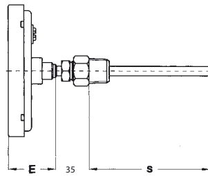
4 - Осевой монтаж
